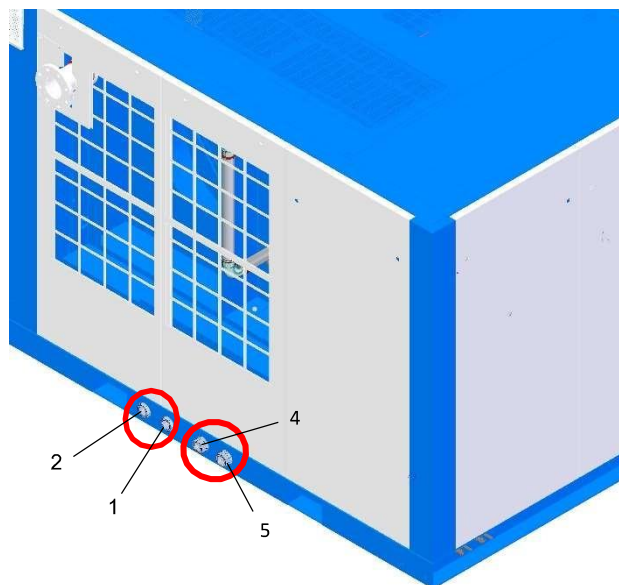
Рис.20: Подключение воды
