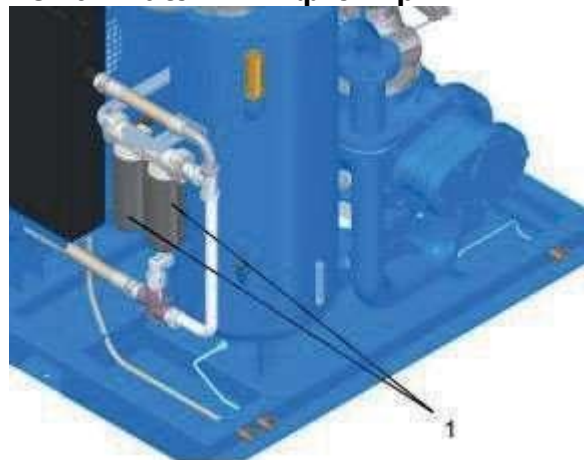
Рис. 14: Масляный фильтр очистки масла
